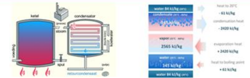
Warmte terugwinning uit condensaat
